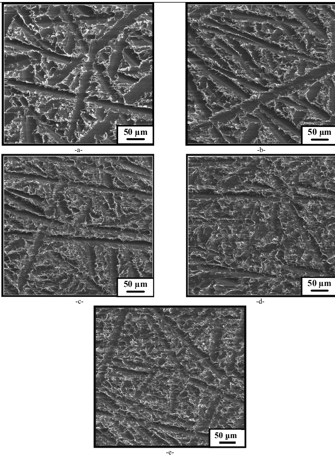
Fig. 11. Superfície produzida na simulação LTM. a- 500 eventos; b- 1000 eventos; c- 1500 eventos; d- 2000 eventos; e- 2500 eventos. Inclinação: 30°, MEV.
