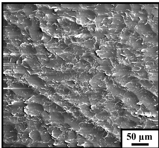
Fig. 5. Superfície obtida na simulação. Área 1\times 1\text{ mm} , 2000 eventos. MEV.
