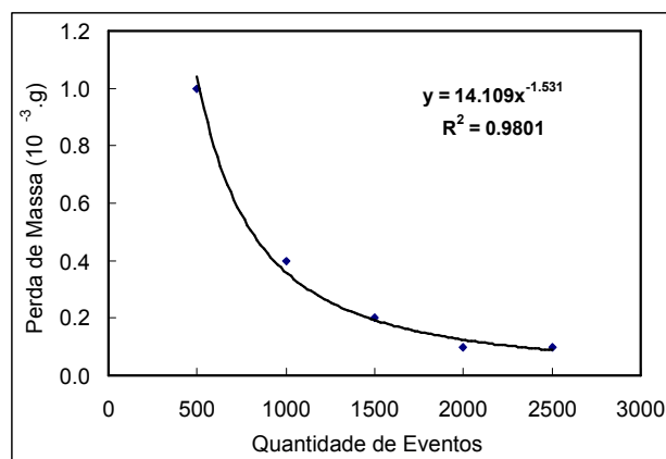
Fig. 8. Perda de massa em função da quantidade de eventos.
