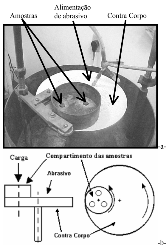
Fig. 1. a- Abrasômetro LTM; b-esquema.
