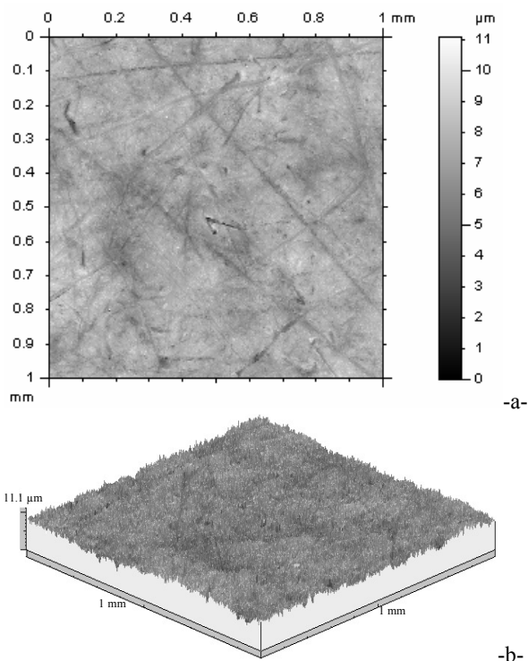
Fig. 4. Interferometria a laser: a- topografia da superfície desgastada; b- topografia em perspectiva.
