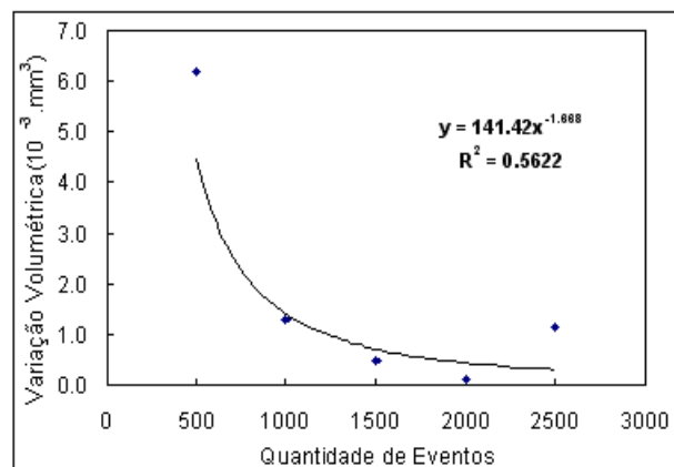
Fig. 9. Variação do volume de material retirado da superfície em função da quantidade de eventos.
