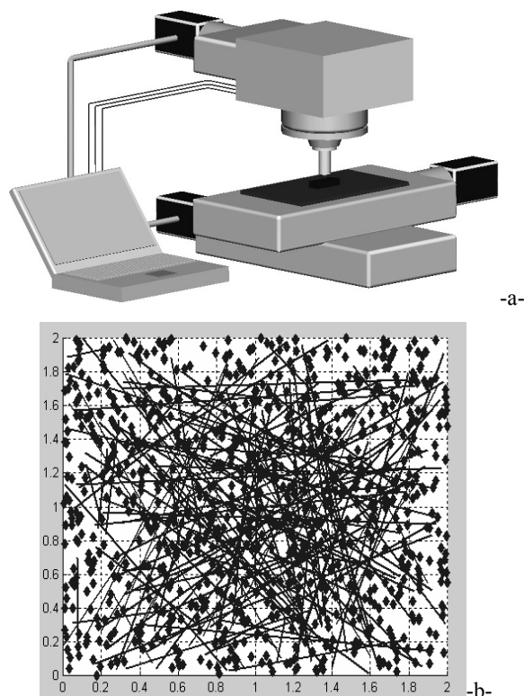
Fig. 2. Simulação LTM. a- esquema; b- área da simulação, representação de 1000 eventos (85% indentações).
