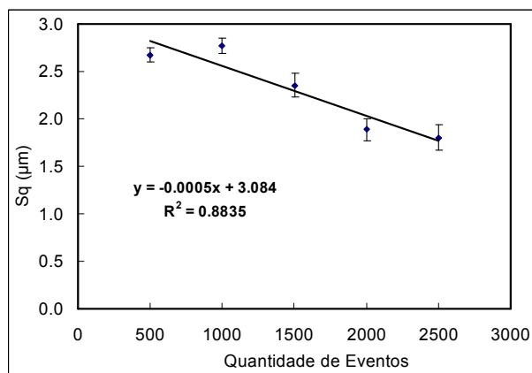
Fig. 10. Rugosidade 'Sq' em função da densidade de eventos.
