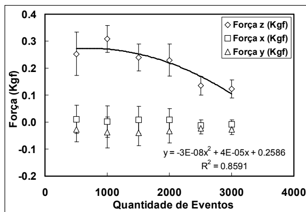
Fig. 7. Componentes da força adquiridas durante todo o ensaio.
