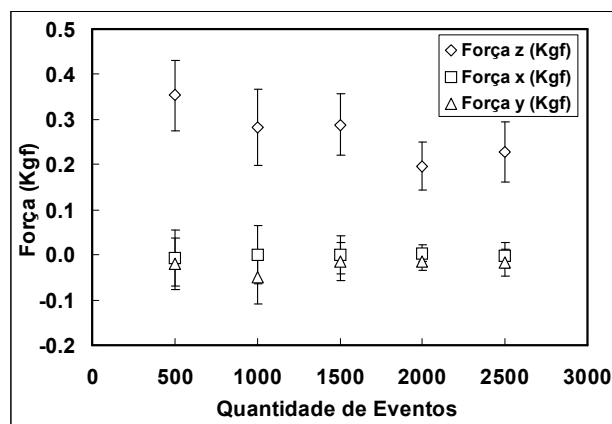
Fig. 12. Componentes da força resultante média em função da quantidade de eventos.
