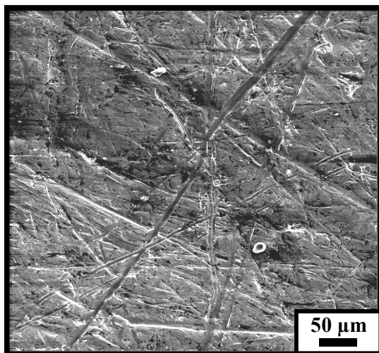
Fig. 3. Superfície desgastada. Inclinação 30°, MEV.
